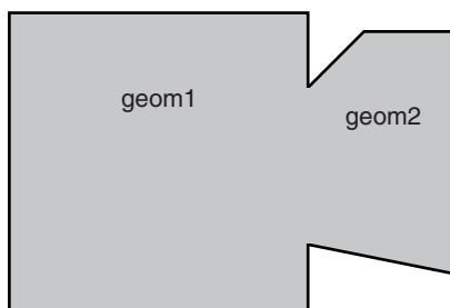
Figure 24–4 SDO_GEOM.SDO_UNION
